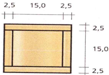
Vista Superior
